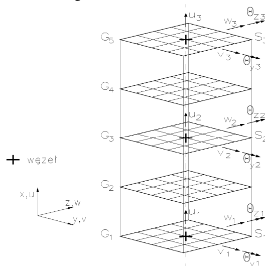
Rys. 3. Trójwęzłowy element pręta z przekrojami wielopunktowymi (elementami FE) z 5 punktami całkowania
